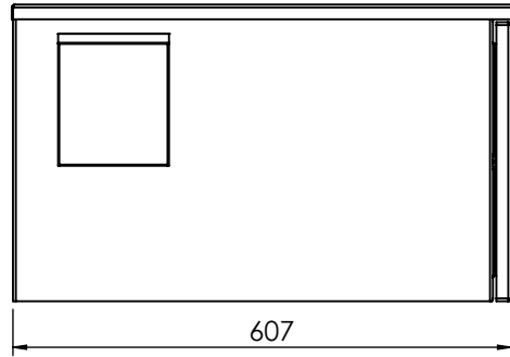
Szafa rack wisząca 6U 60x60
